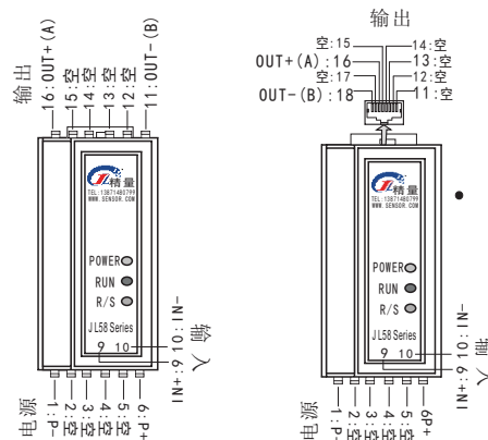
免螺丝端子接线图
