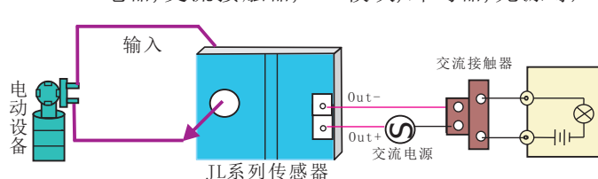
示例四: 结合接触器间接控制交直流负载 (比如: 继电器, 交流接触器, PLC模块, 蜂鸣器, 光源等)
