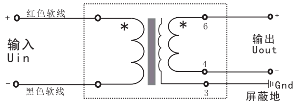
安装使用说明: 输入为引线; 4, 6脚为输出; 3脚为屏蔽; 输入引线红色标记与6脚为同名端。
