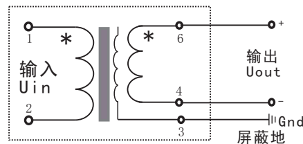
安装使用说明: 1, 2脚为输入; 4, 6脚为输出; 3脚为屏蔽; 1脚与6脚为同名端。
